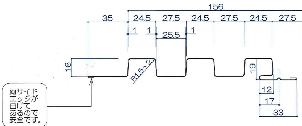
断面図 S=1:2
